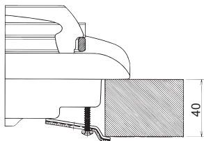
Position der Haken für Arbeitsplatten H=40mm
