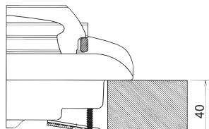
Posizione gancio per top H=40mm
