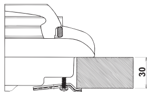
Position der Haken für Arbeitsplatten H=30mm
