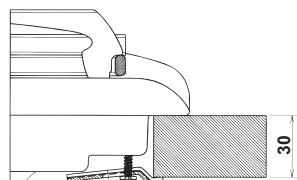
Position du crochet pour top H=30mm
