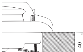
Posición del gancho para superficies H=40mm
