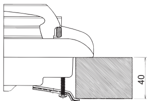
Stand haak voor keukenblad H=40mm
