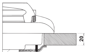
Position du crochet pour top H=20mm
