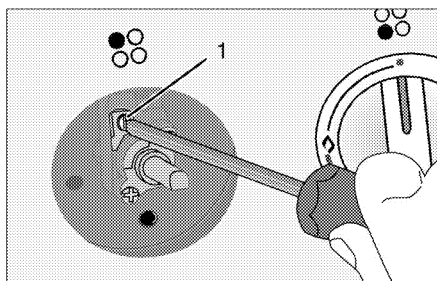
1 Stelschroef gasdebiet
